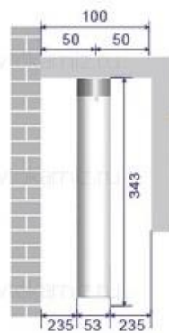
Установка одного мотора
