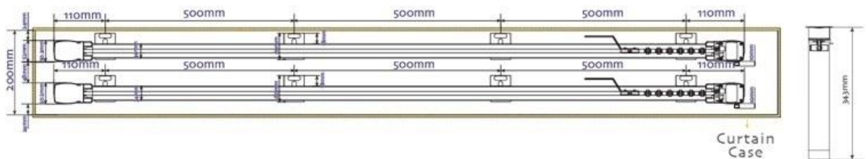
Установка двух алюминиевых профиля к потолку
